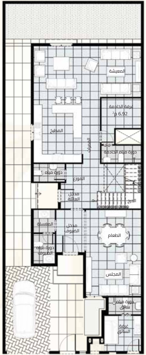
الدور الأرضي 150 م²
