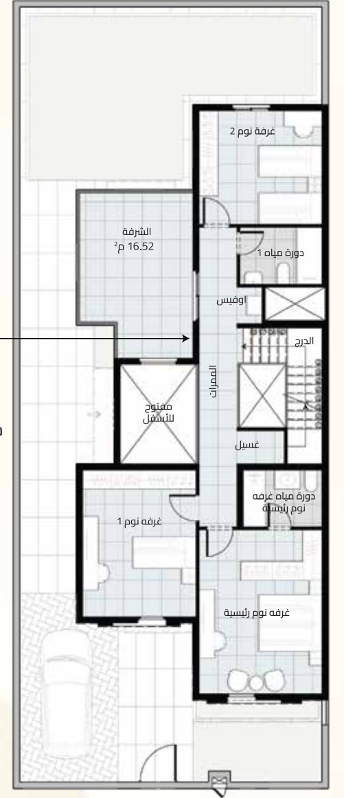
الدور الأول 96م²
