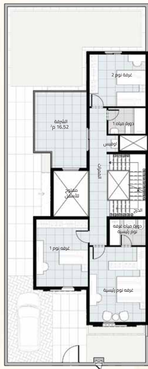
الدور الأول 96 م 2
